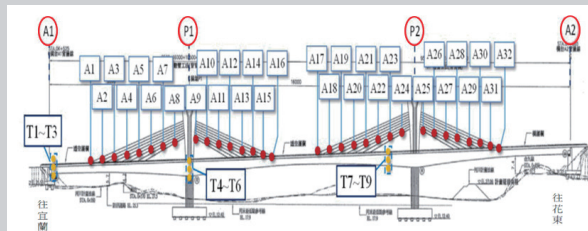
圖 7. 橋梁儀器配置示意圖
